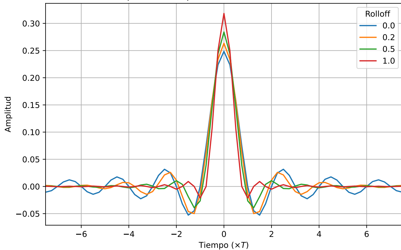
Respuesta al Impulso del Raíz Coseno Realzado
